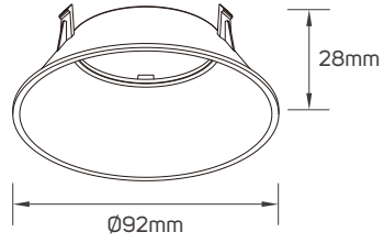
613115 - 613116 - 613117 - Reflector
