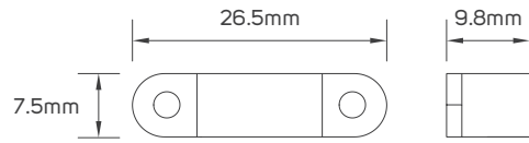
613555 - Clips
